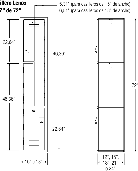
Vista delantera
